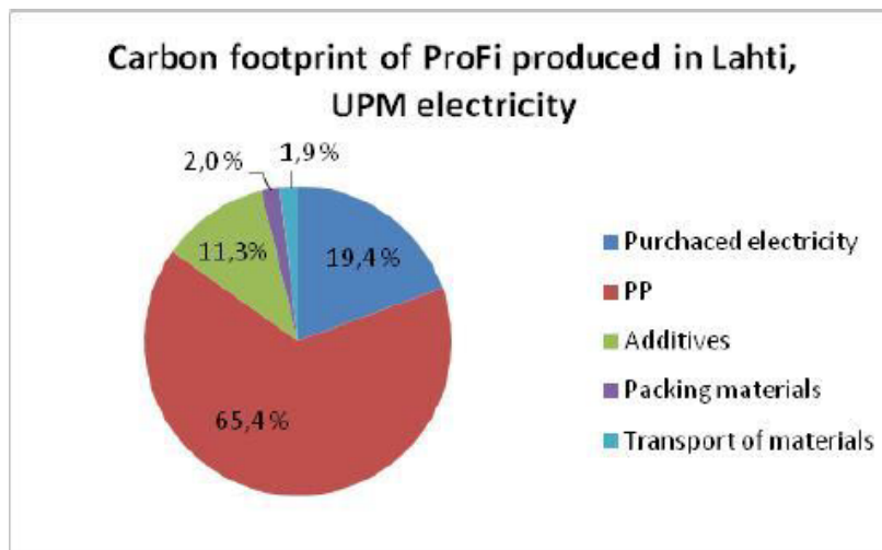
Figur 3: Carbon-footprint WPC produkten UPM ProFi (kilde: VTT Research Report VTT-R -02591-11.2011)
